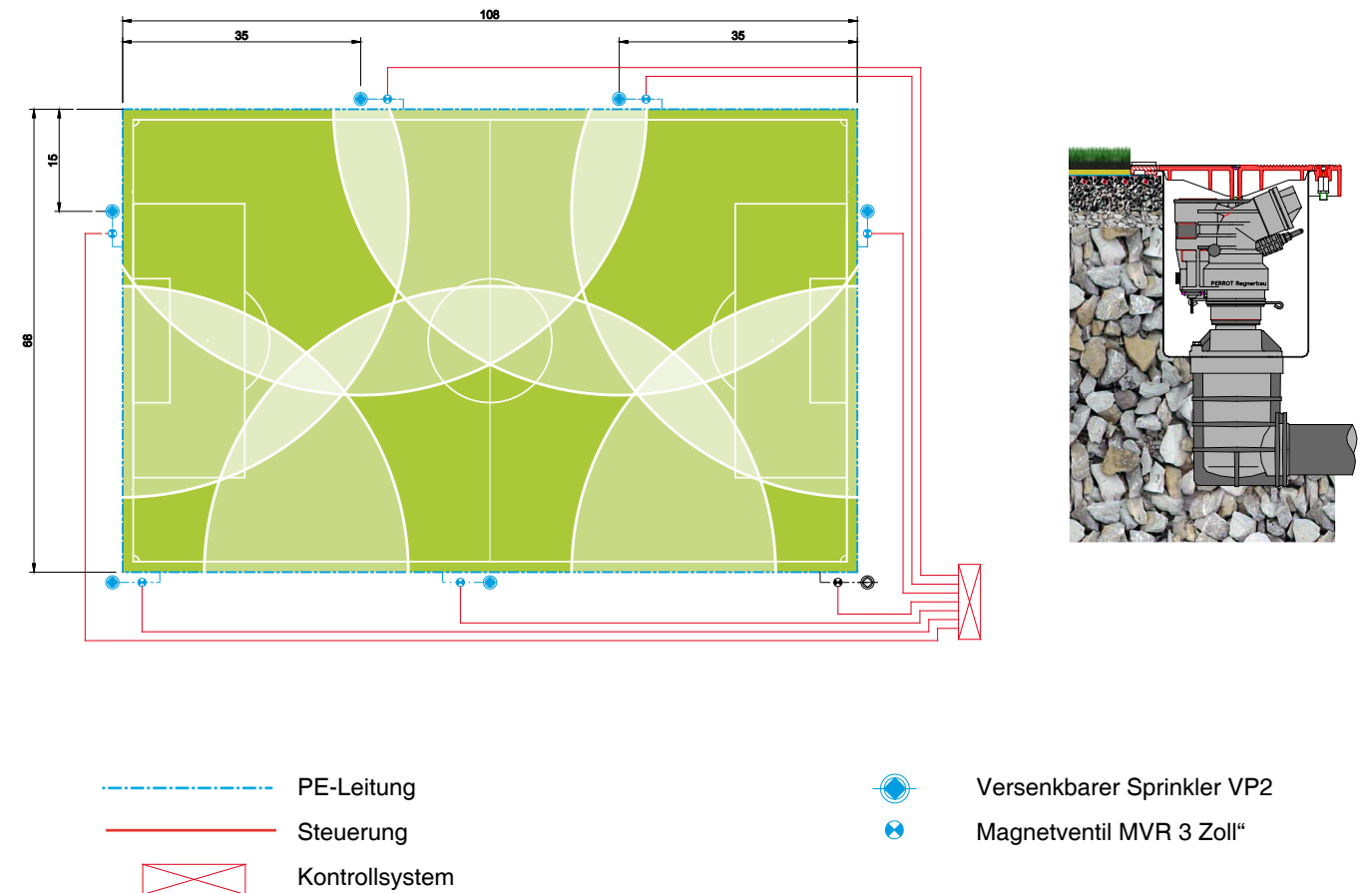
Schema einer Bewässerungsanlage ausserhalb der Spielfeldzone
