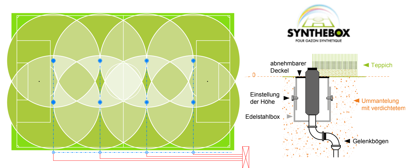
Schema einer Bewässerungsanlage in der Spielfeldzone Synthebox
